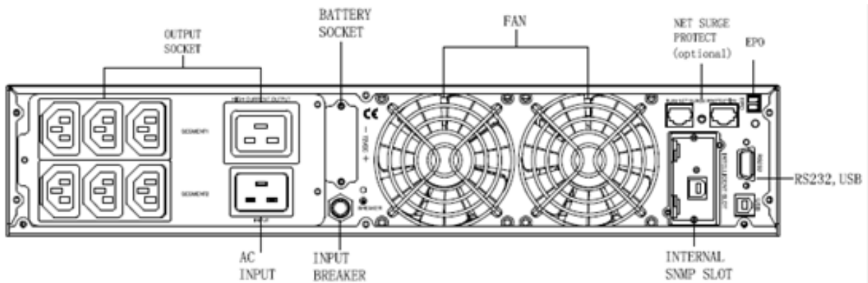
Рис.3 Задняя панель 2kVA/3kVA
