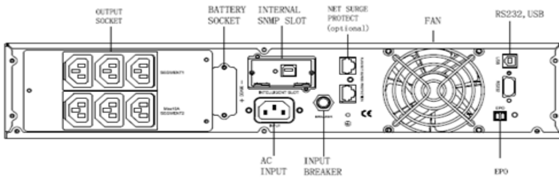
Рис.2 Задняя панель 1 kVA / 1,5 kVA
