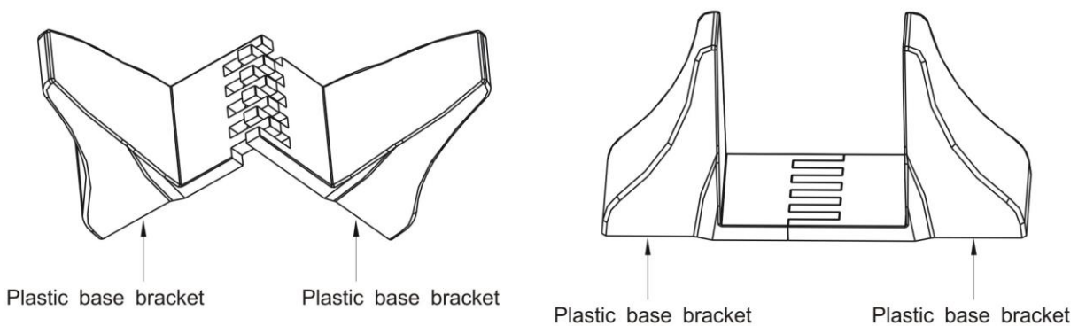
Рис.8 Пластмассовый крепеж
