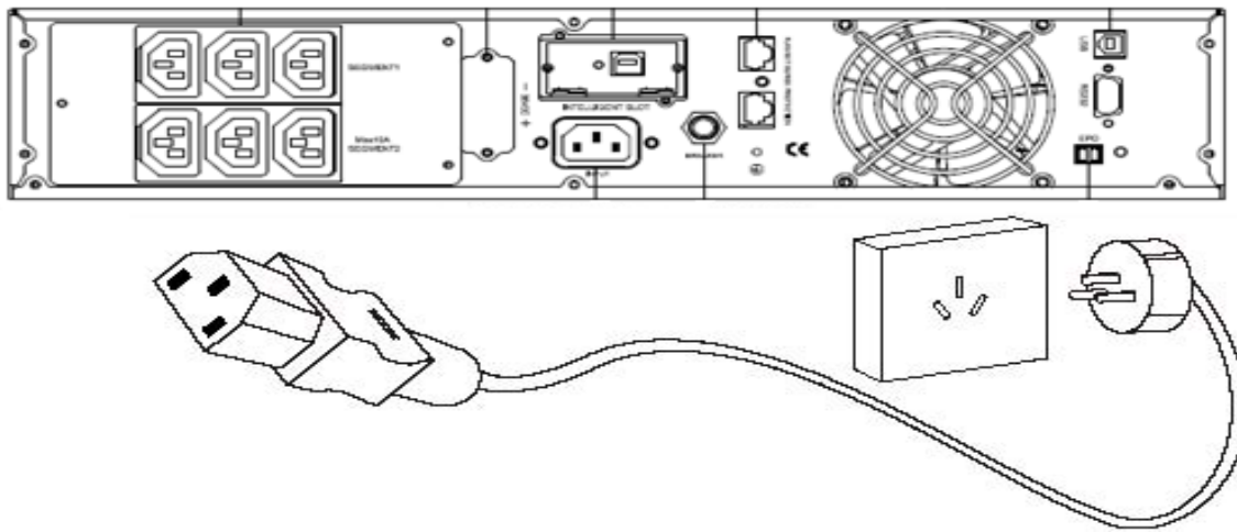
Рис. 5 Подключение на входе
